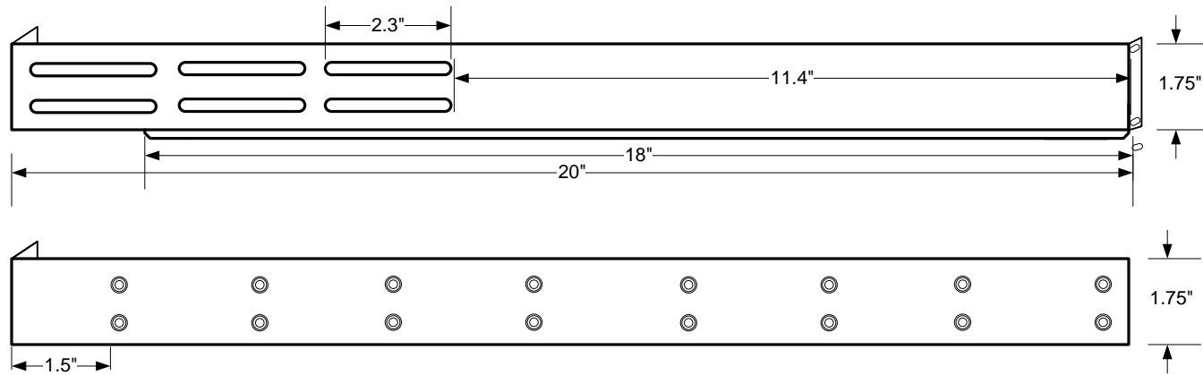
MOUNTING EDGE SIDE
